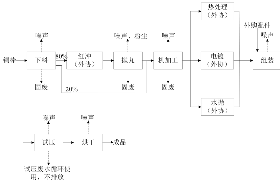
图 2-1 阀门生产工艺流程图
